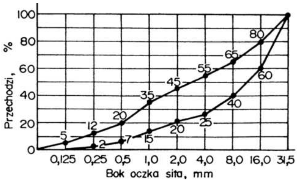
Rysunek 2. Graniczne krzywe uziarnienia kruszywa do podbudowy z betonu od 0 do 63 mm.
